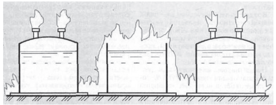
Зураг 1. – Мазут хадгалж буй резервуарын гал түймрийн үед шатах шингэний цацагдах үеийн зураглал
