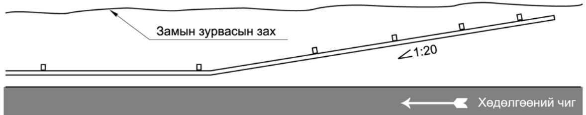
G.3-р зураг – Ойртолтын шугаман хашилтыг байрлуулах бүдүүвч
