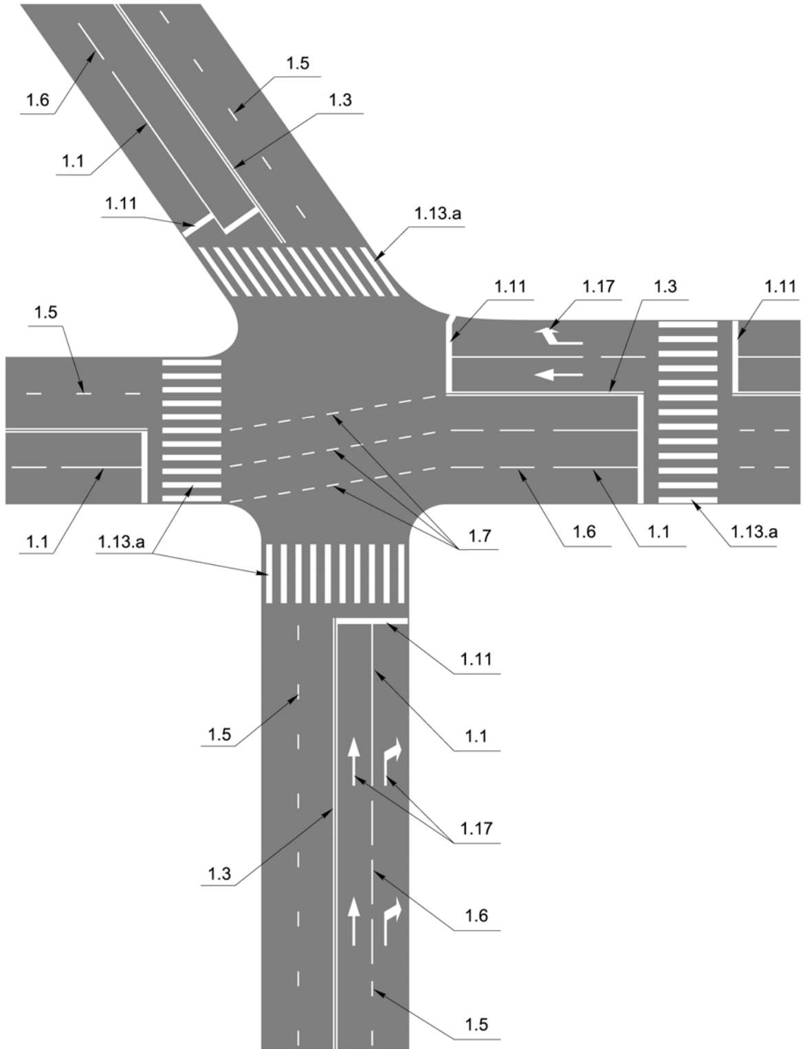
Е.4-р зураг – Зохицуулдаг уулзварт тэмдэглэл тавих жишээ
