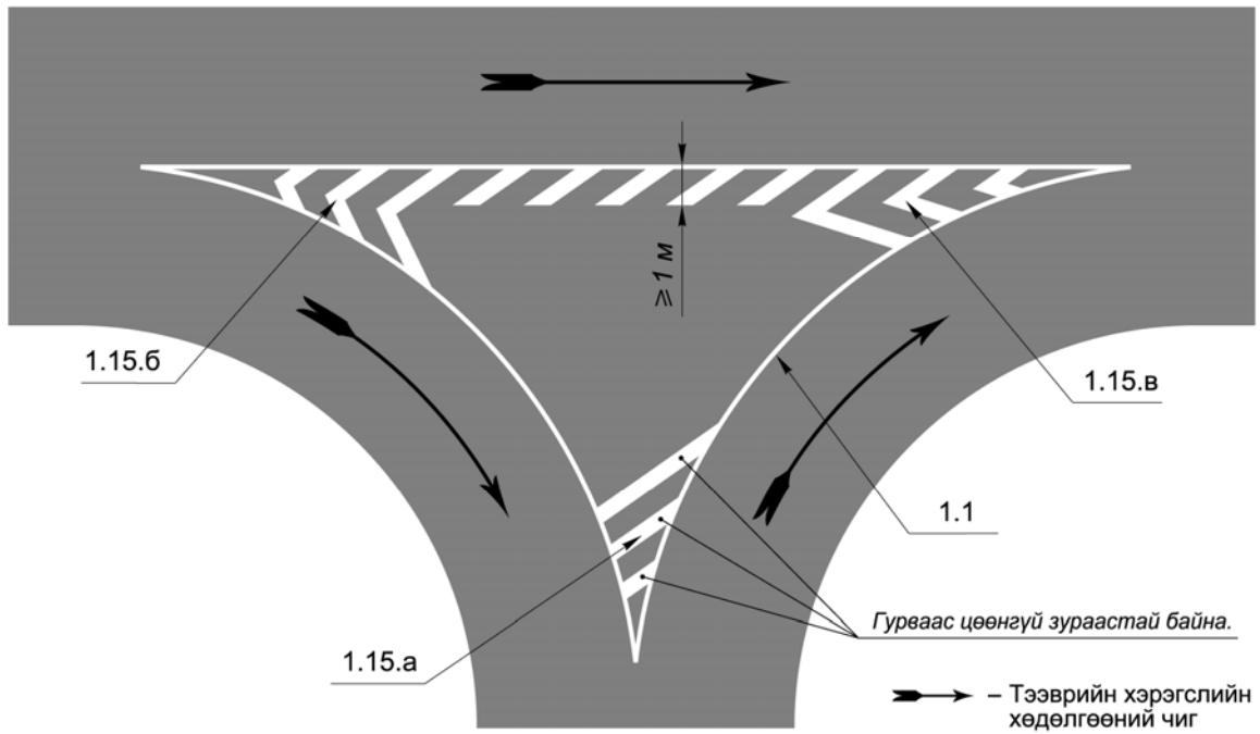
Е.6-р зураг – Чиглүүлэгч арлыг тэмдэглэх жишээ
