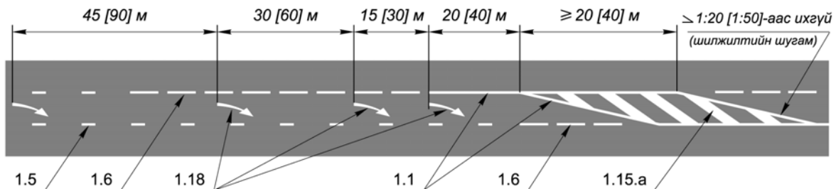
Е.3-р зураг – Нэг чиг дэх хөдөлгөөний эгнээний тоо хасагдах хэсэгт тэмдэглэл тавих жишээ
