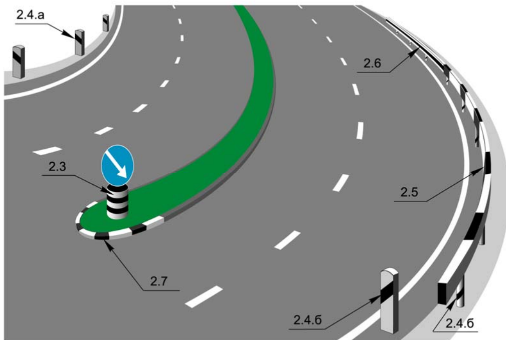
Е.16-р зураг – 2.3–2.7 тэмдэглэлүүдийг хэрэглэх жишээ
