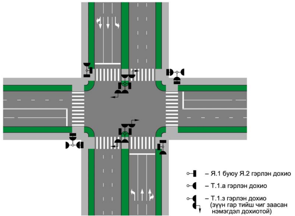
F.3-р зураг – Уулзварт гэрлэн дохиог байрлуулах бүдүүвч
