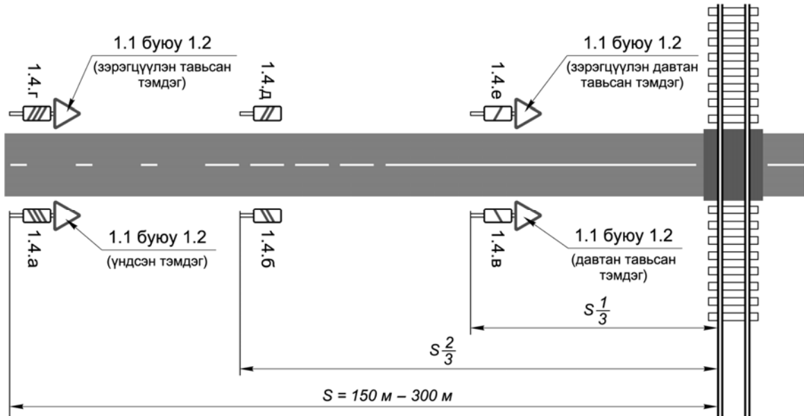
D.3-р зураг – 1.4.а–1.4.е тэмдгийг байрлуулах бүдүүвч
