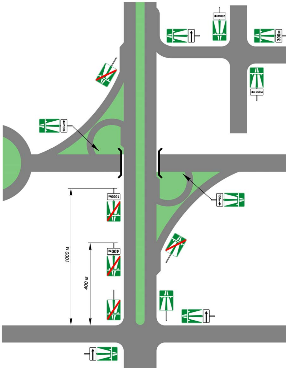
D.5-р зураг – 5.1 ба 5.2 тэмдгийг байрлуулах жишээ
