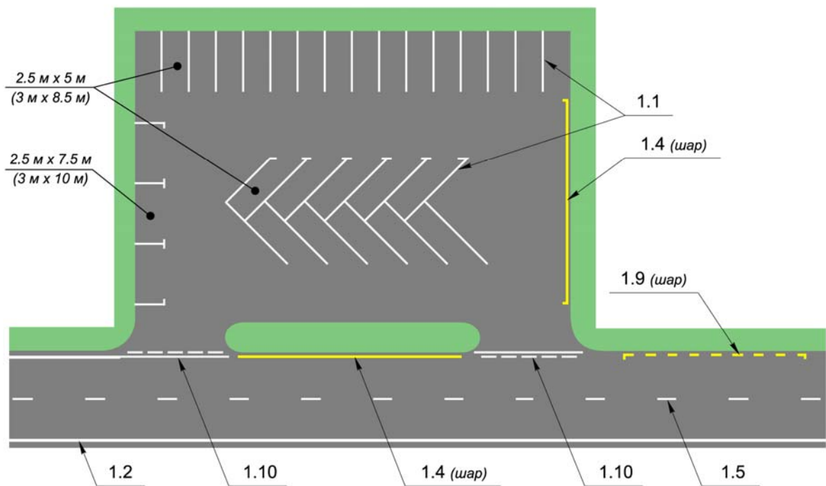
Е.7-р зураг – Тээврийн хэрэгслийн зогсоолын талбай дээр тэмдэглэл тавих жишээ
