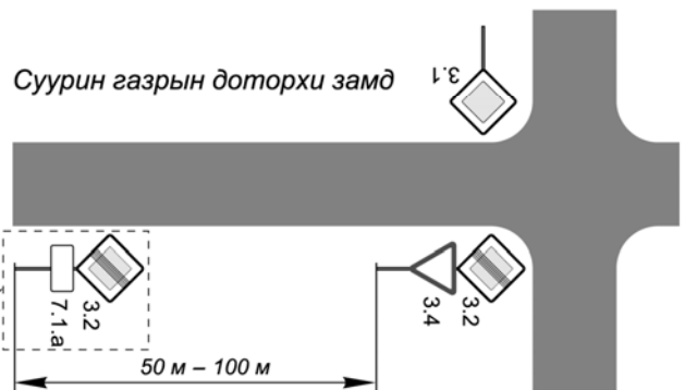
D.4-р зураг – Дарааллын тэмдгийг байрлуулах жишээ
