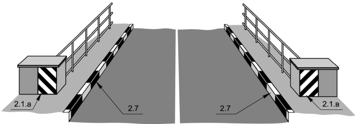
Е.15-р зураг – 2.1.а, 2.1.в, 2.7 тэмдэглэлийг хэрэглэх жишээ
