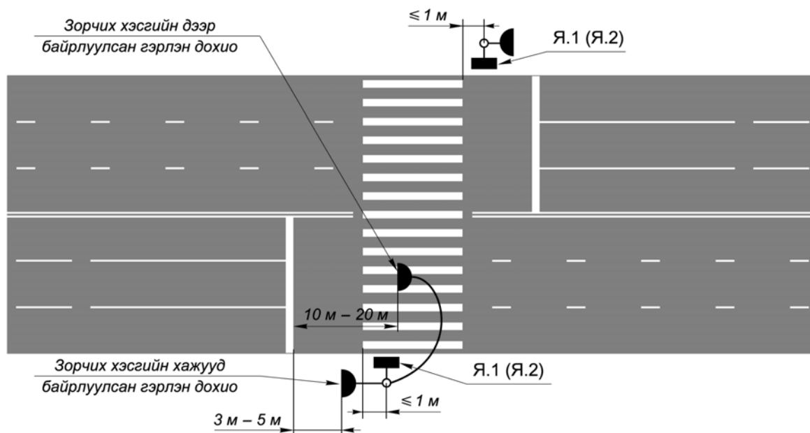
F.2-р зураг – Явган хүний гарц дээр гэрлэн дохиог байрлуулах бүдүүвч
