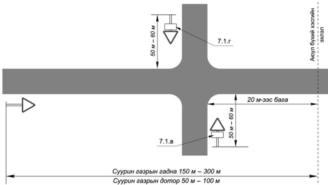
D.2-р зураг – Анхааруулах тэмдгийг байрлуулах жишээ
