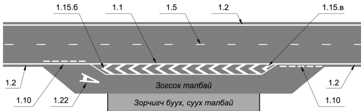
Е.9-р зураг – Чиглэлийн тээврийн хэрэгслийн буудлын талбайг тэмдэглэлээр тусгаарлах жишээ
