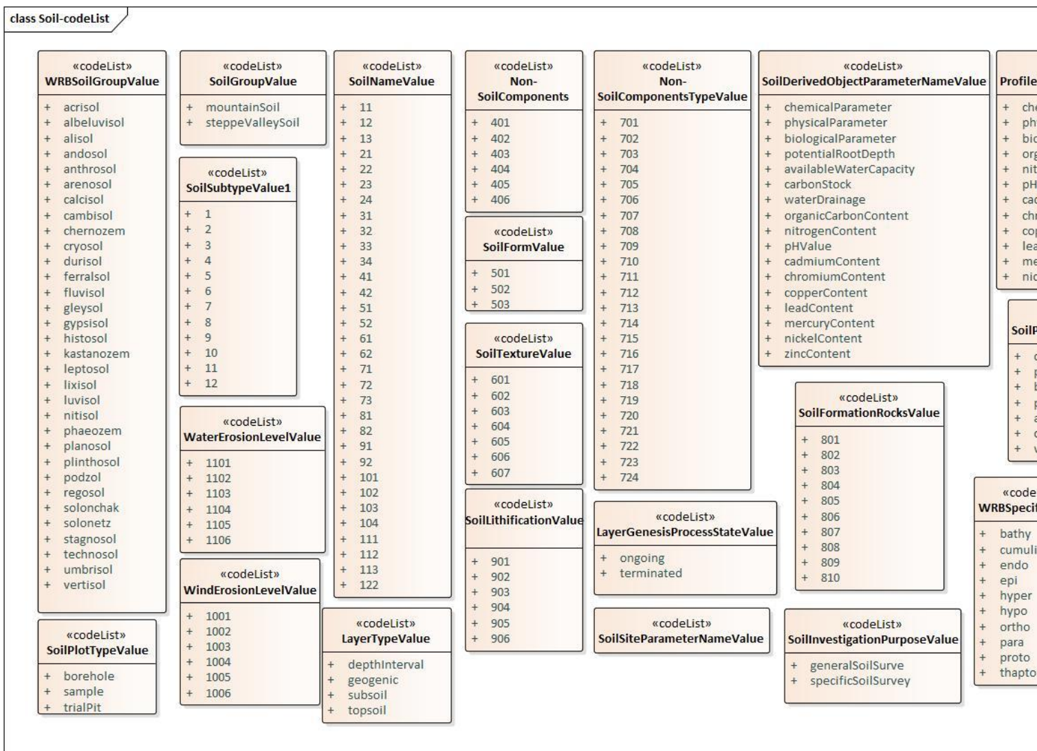
С.4-р зураг UML диаграмм: Soil-ний кодын жагсаалтын схем
