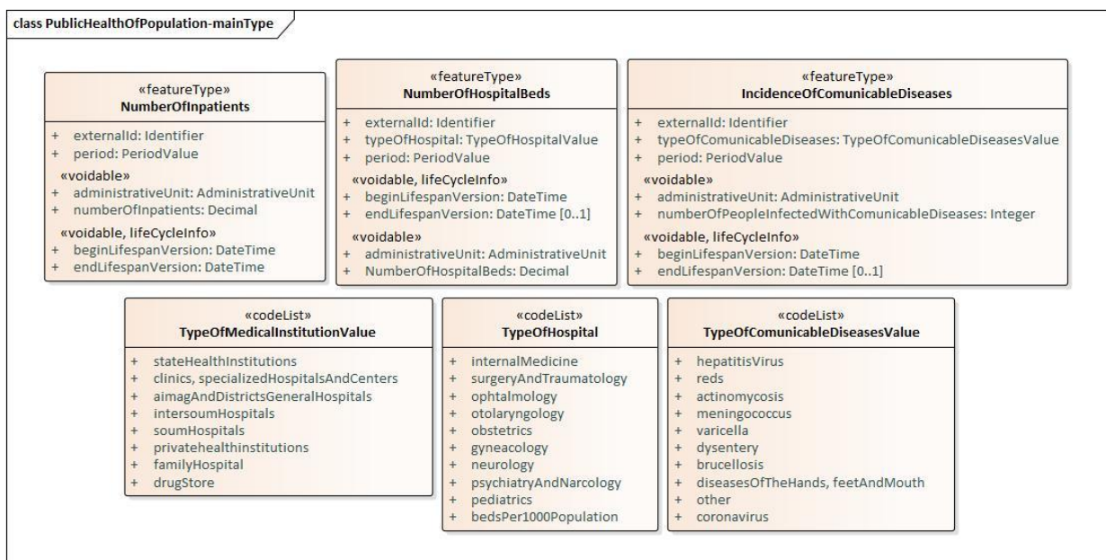
С.9-р зураг - UML диаграмм: Эрүүл мэнд багцын ерөнхий хүснэгт
