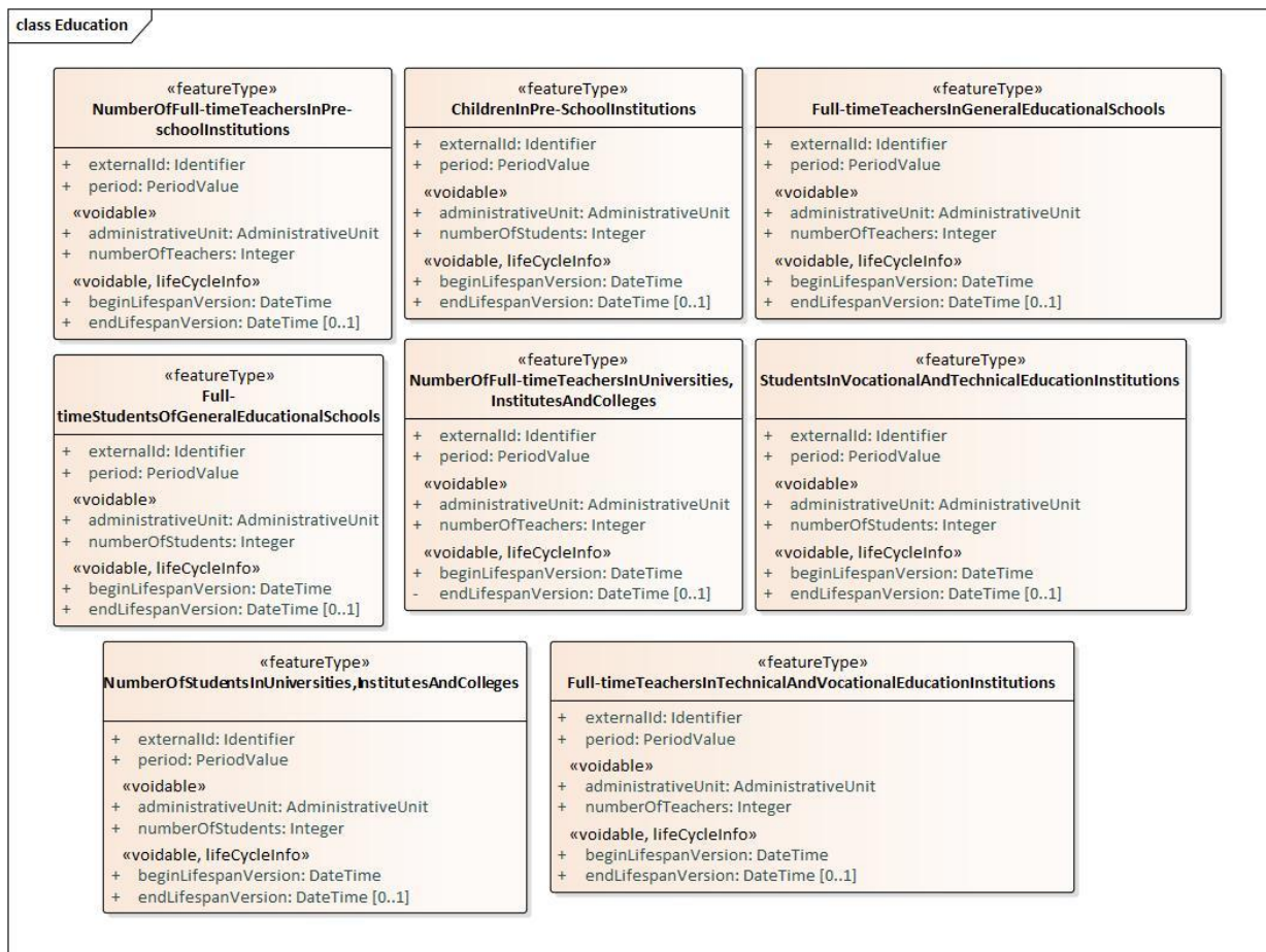
С.11-р зураг - UML диаграмм: Боловсрол багцын ерөнхий хүснэгт
