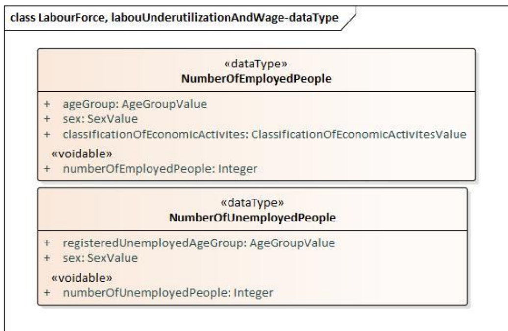
C.5-р зураг - UML диаграмм: Хөдөлмөр эрхлэлт, хөдөлмөрийн дутуу ашиглалт, дундаж цалин багцын өгөгдөл төрөл
