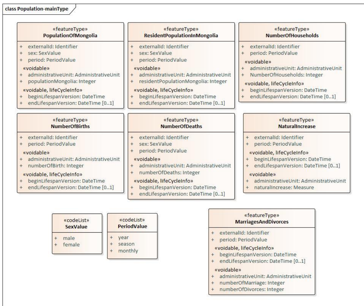
C.2-р зураг - UML диаграмм: Хүн ам багцын ерөнхий хүснэгт
