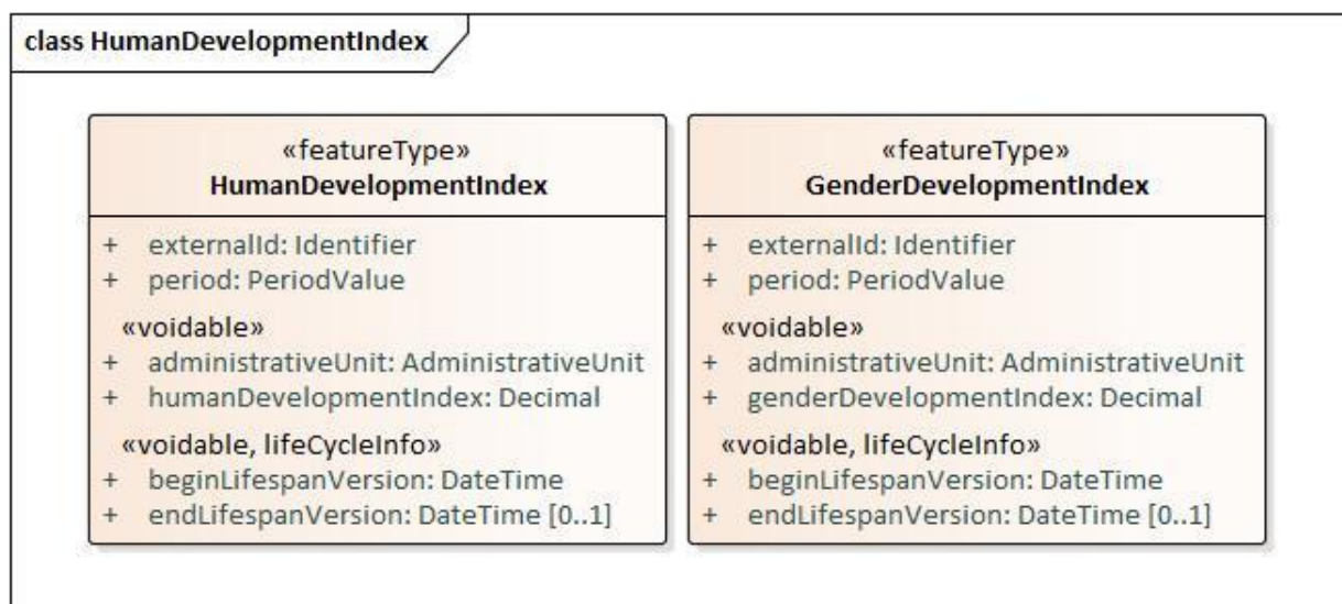
С.11-р зураг - UML диаграмм: Хүний хөгжлийн индекс багцын ерөнхий хүснэгт
