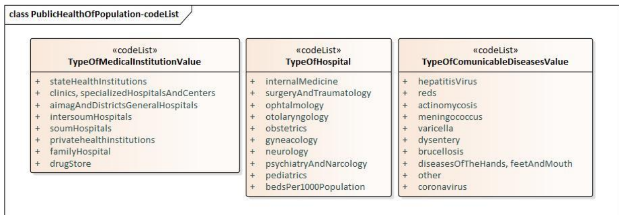
С.10-р зураг - UML диаграмм: Эрүүл мэнд багцын кодын жагсаалт
