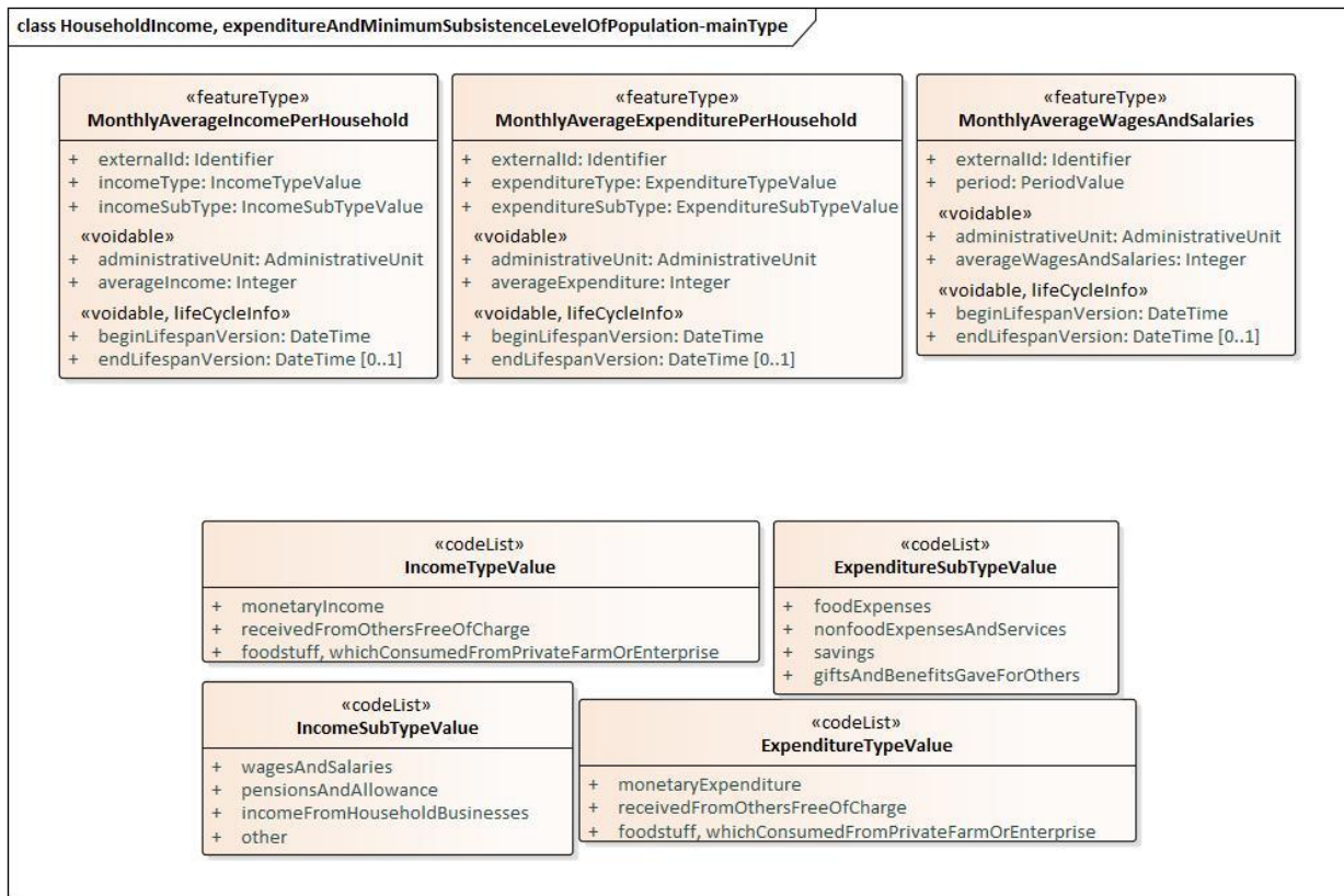
С.7-р зураг - UML диаграмм: Ядуурал, өрхийн орлого, зарлага, дундаж хэрэглээ багцын ерөнхий хүснэгт
