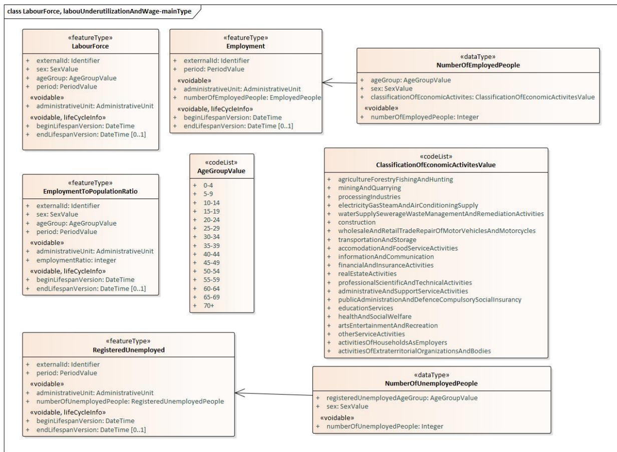
C.4-р зураг - UML диаграмм: Хөдөлмөр эрхлэлт, хөдөлмөрийн дутуу ашиглалт, дундаж цалин багцын ерөнхий хүснэгт
