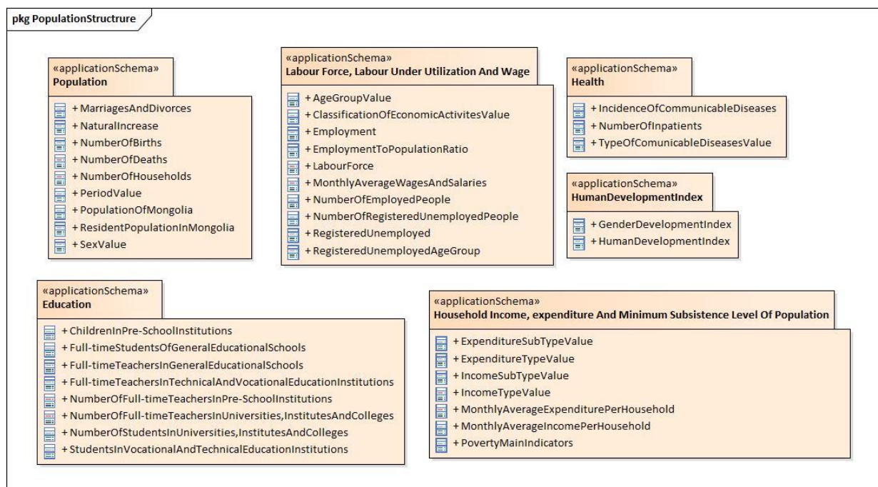
С.1-р зураг - UML диаграмм: Хүн ам, нийгмийн салбарын мэдээллийн орон зайн өгөгдлийн үзүүлэлт – Үндсэн төрлүүдийн тойм
