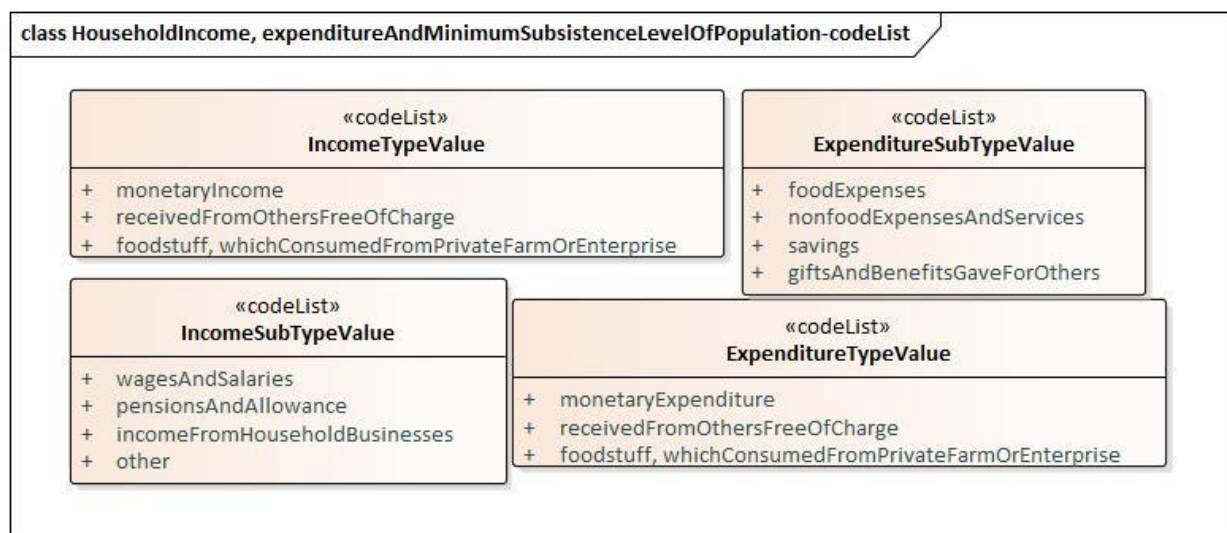
С.8-р зураг - UML диаграмм: Ядуурал, өрхийн орлого, зарлага, дундаж хэрэглээ багцын кодын жагсаалт
