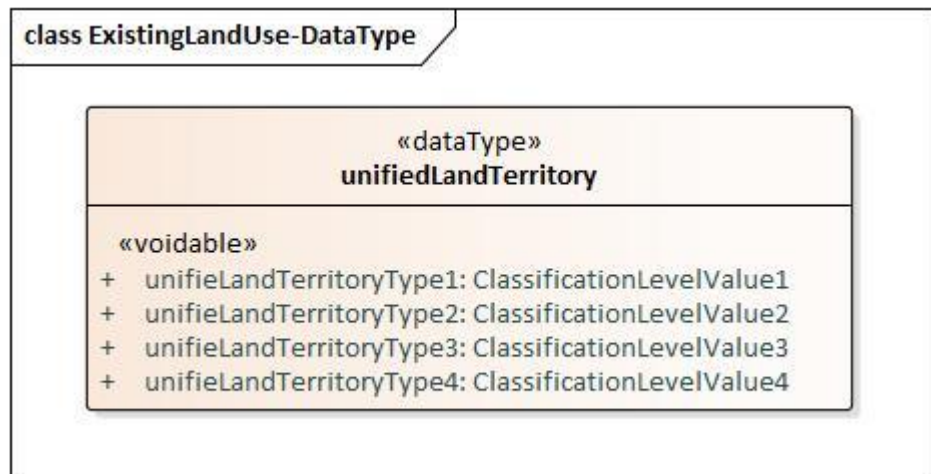
С.3-р зураг UML диаграмм: Existing land use-ийн өгөгдөл төрөл
