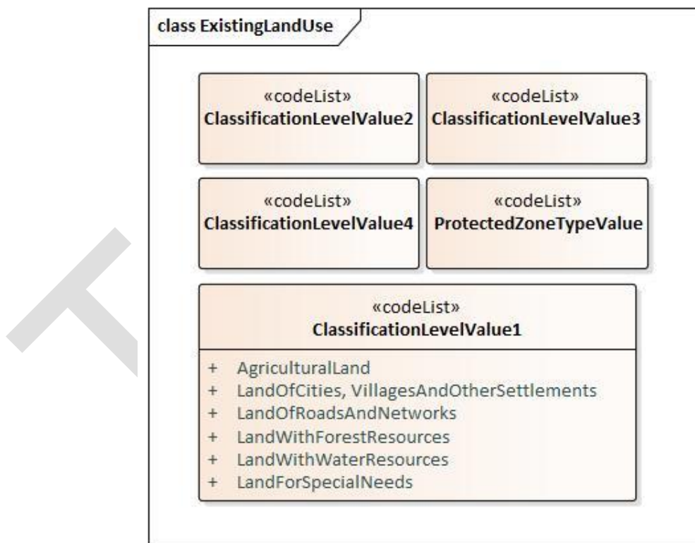
С.5-р зураг UML диаграмм: Existing land use-ийн кодын жагсаалтын схем
