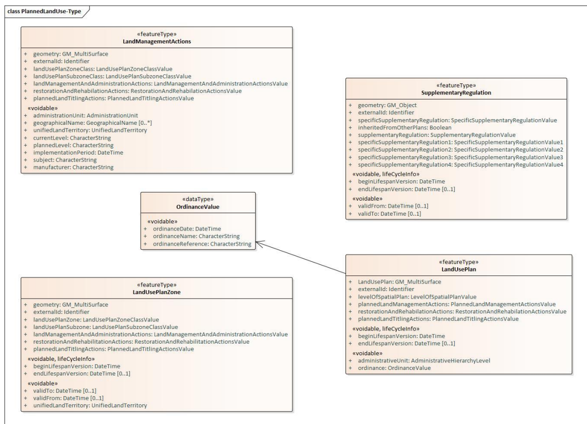
С.5-р зураг UML диаграмм: Planned land use-ийн ерөнхий схем
