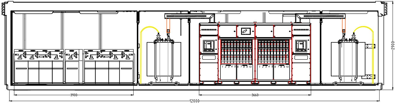
Байгууламжийн дотор огтлол /ургаас/
