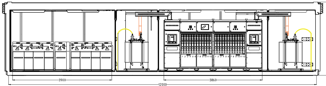
Тэнхлэгээс тэнхлэг хоорондох хэмжээ
