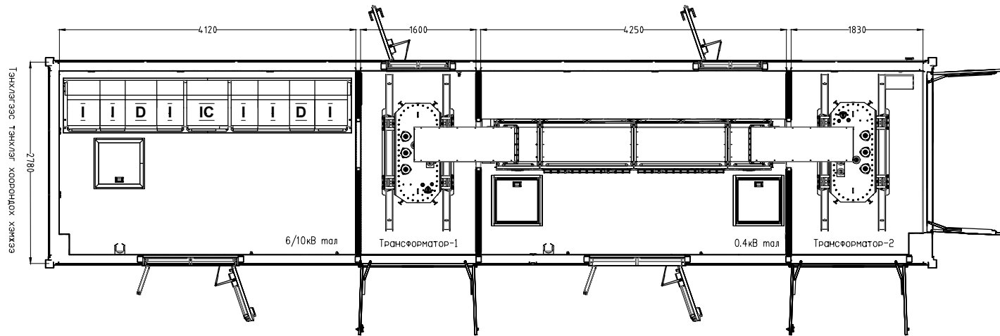
Багаууламжийн дотор огтлол /гээрээс/
