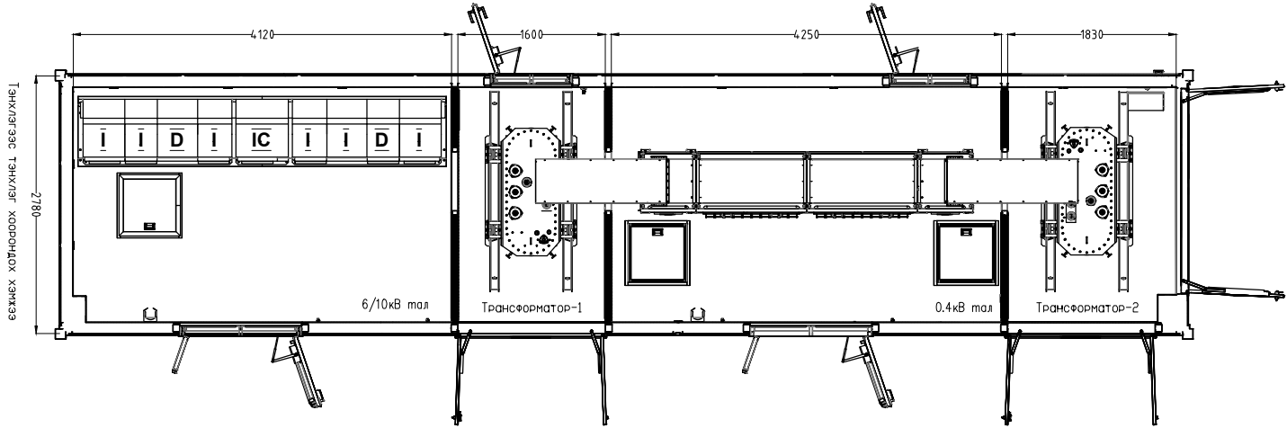
Байгууламжийн дотор огтлол /гээрээс/
