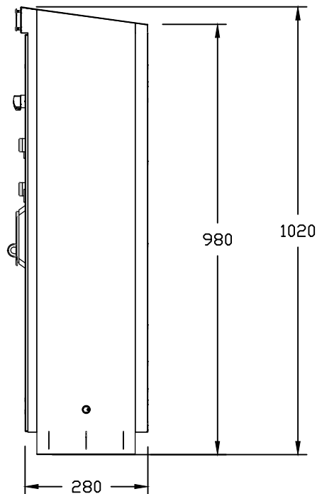
Хажуу тал
