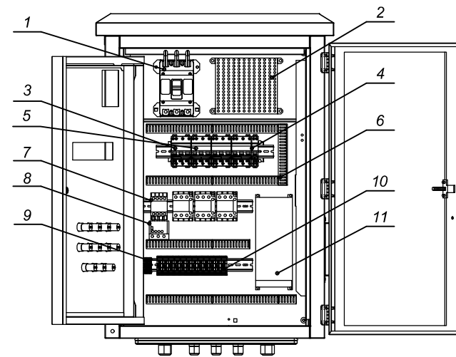
Дотор тоноглол
