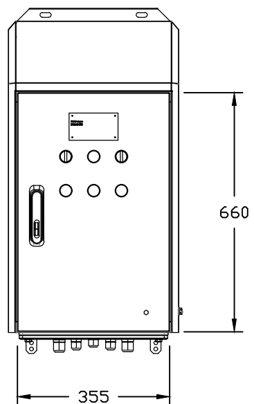
Нүүрэн тал
