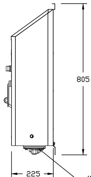
Хажуу тал
