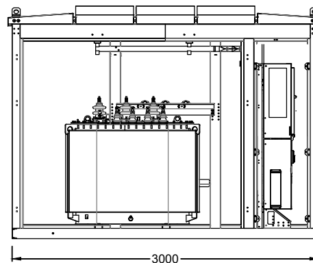
Трансформатор тал-Б
