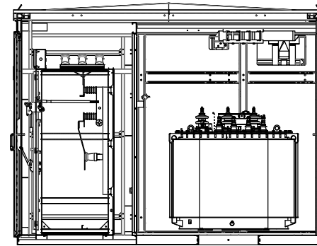
Трансформатор тал-Б
