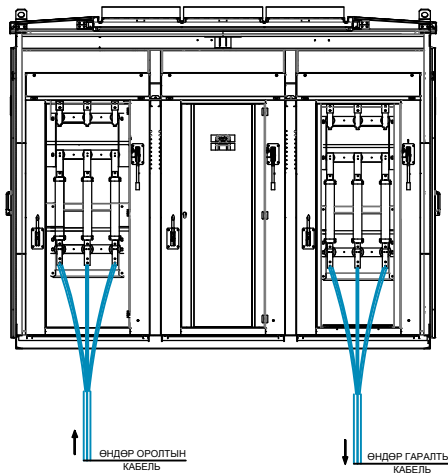
Дунд хүчдэл тал-В
