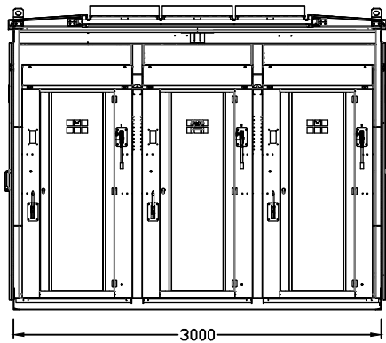
Дунд хүчдэл тал-В
