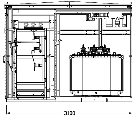
Трансформатор тал-Б
