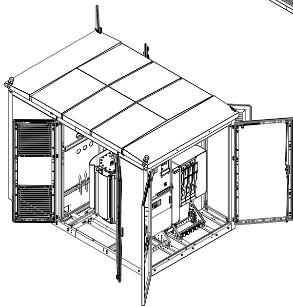
ИТД-загвар PE.Z-630D-RM6 харагдах байдал
