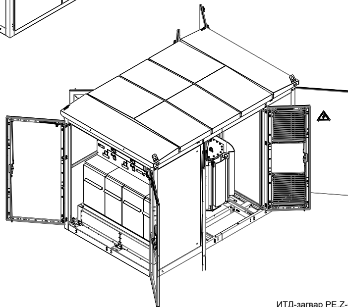
ИТД-загвар PE.Z-630D-RM6 харагдах байдал
