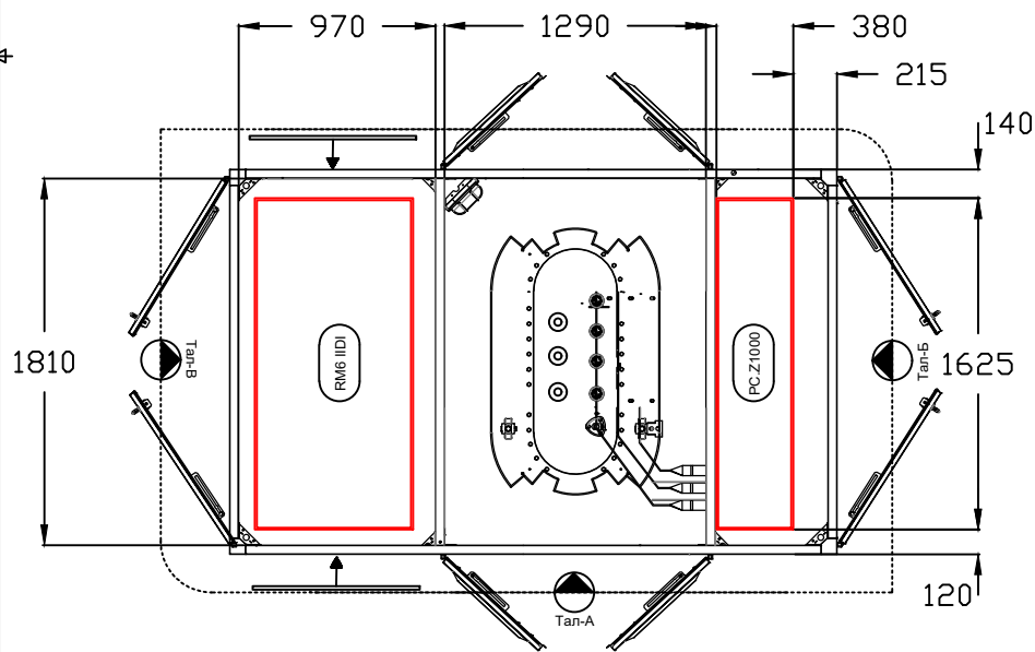
План: тасалгааны байгуулалт хэмжээ
