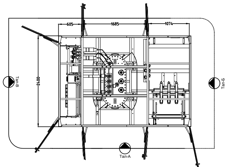
План: тасалгааны байгуулалт хэмжээ
