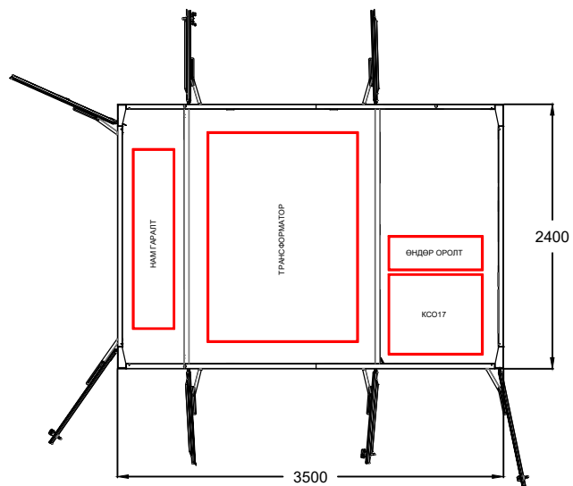
План: Кабель оролт гаралтын нүхний хэмжээ
