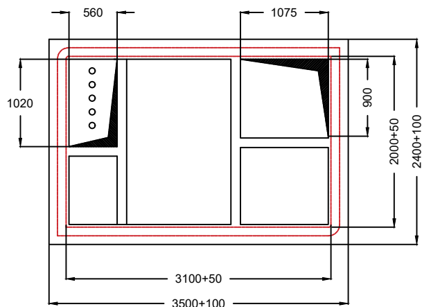
План: Кабель оролт гаралтын нүхний хэмжээ
