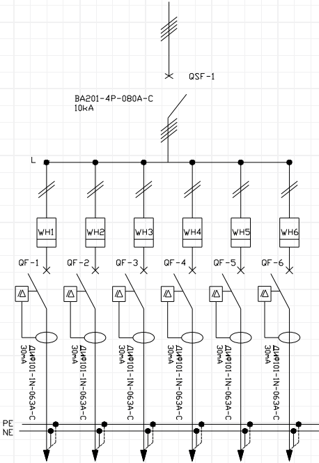
ProCube.T6-M • Ерөнхий автомат • Тоолуур • Гаралтын дифференциал автомат
