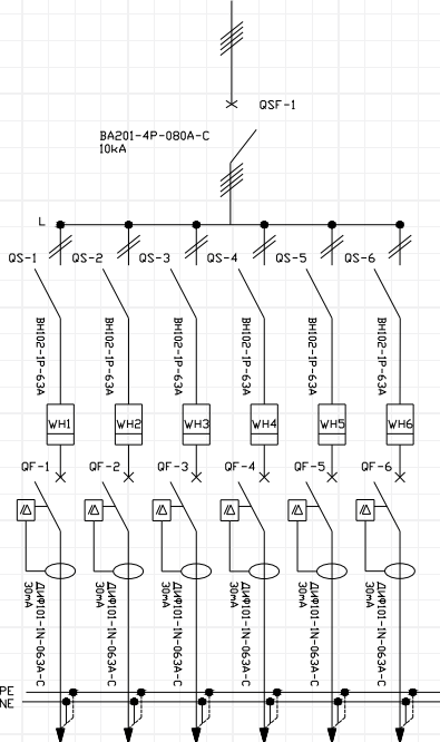
ProCube.T6-MR • Ерөнхий автомат • ачаалал таслагч • Тоолуур • Гаралтын дифференциал автомат
