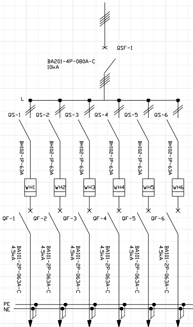
ProCube.T6-R • Ерөнхий автомат • ачаалал таслагч • Тоолуур • Гаралтын энгийн автомат
