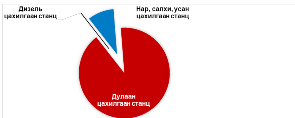
График 22. Цахилгаан эрчим хүчний нийт хэрэглээ
