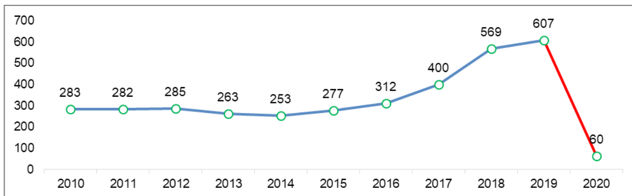
График 24. 2010-2020 оны аялал жуулчлалын салбарын орлого (сая ам. доллар)
