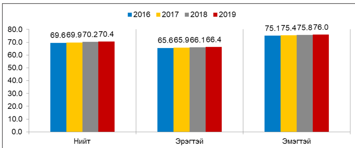
График 25. Хүн амын дундаж наслалт
