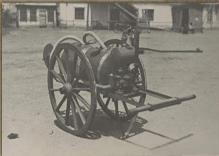
100 литрийн багтаамжтай, мориор чирдэг, гар насос бүхий усан хөөргийг 1922-1925 хүртэл гал унтраахад ашиглаж байжээ.
