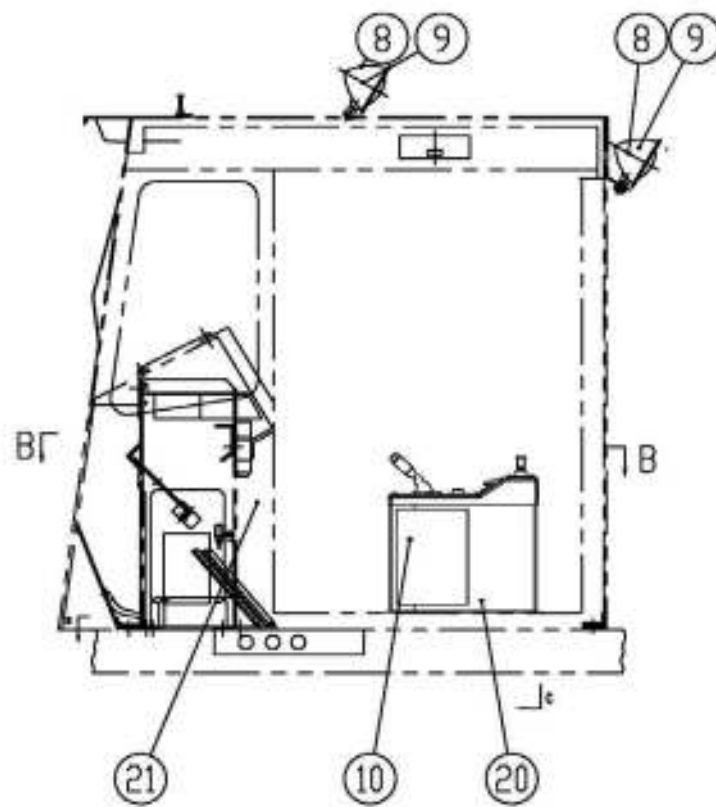
B-B
